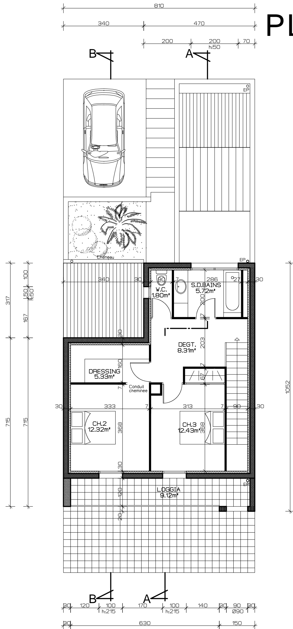
PLAN ETAGE
